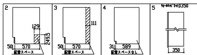
レイアウト展開図A
