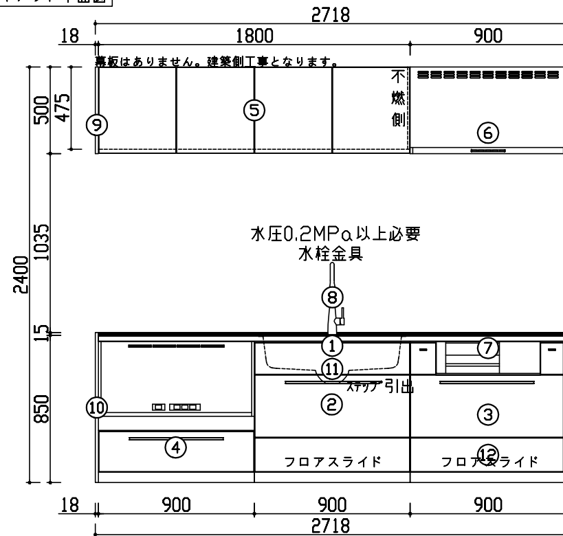
レイアウト展開図A
